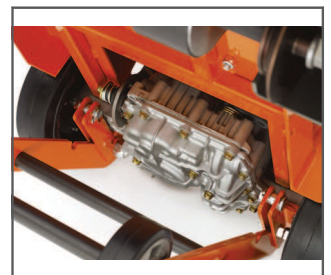
NIEZALEŻNY NAPĘD Niezależny napęd różnicowy eliminuje potrzebę użycia mechanizmu napędowego tylnych kół i związanego z tym ich większego zużycia. Jego obsługa i konserwacja są bardzo proste.
