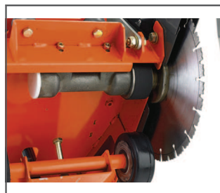
OPTYMALNE PRZEKAZYWANIE MOCY NA TARCZĘ Udoskonalony układ napinania pasa zapewnia stałe napięcie bez potrzeby ponownej regulacji, dając optymalną wydajność i zwiększając trwałość pasa.
